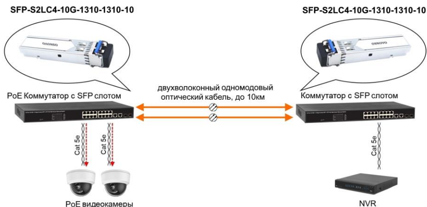
Рис.5 Типовая схема подключения модуля SFP-S2LC4-10G-1310-1310-10
