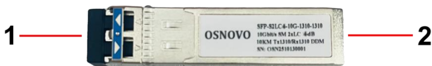
Рис.2 Разъемы SFP модулей SFP-S2LC4-10G-1310-1310-3 и SFP-S2LC4-10G-1310-1310-10
