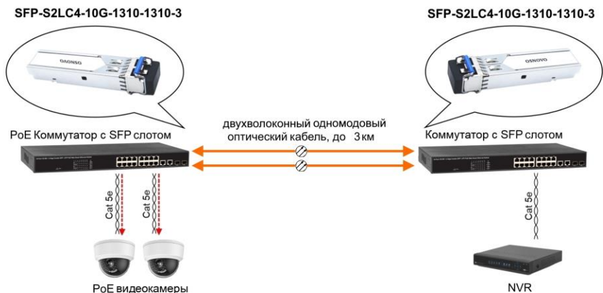
Рис.4 Типовая схема подключения модуля SFP-S2LC4-10G-1310-1310-3
