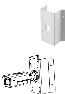
F-AY10004 DS-1276ZI-SUS Кронштейн для установки на угол
