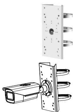
F-AY10003 DS-1275ZI-SUS Кронштейн для установки на столб (стойку)
