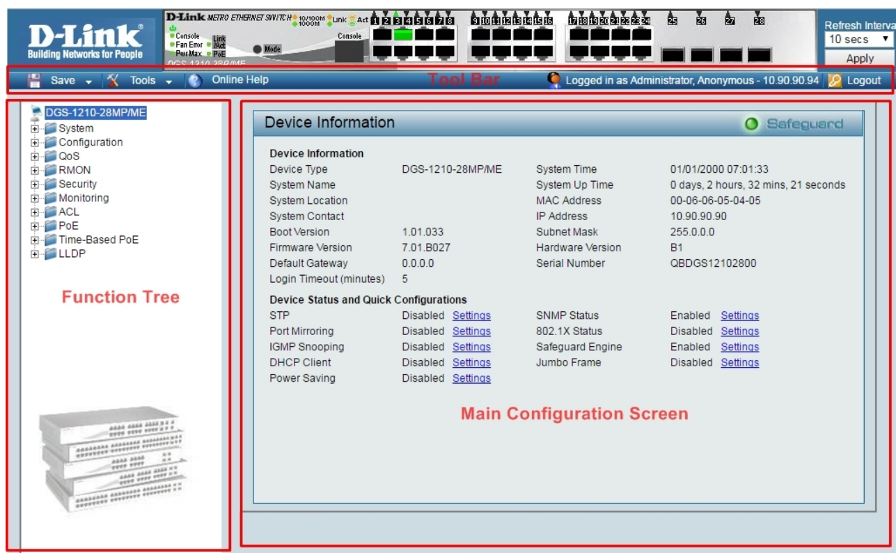
Рисунок 4.3 — Главное окно Web-интерфейса
