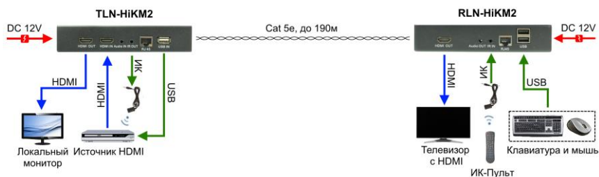
Рис.7 Схема подключения комплекта TLN-HiKM2+RLN-HiKM2 в режиме «точка-точка»
