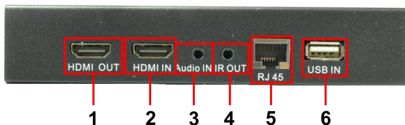
Рис. 3 Передатчик TLN-HiKM2, разъемы и индикаторы на задней панели
