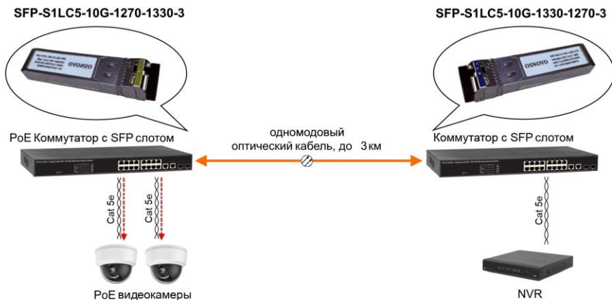
Рис.4 Типовая схема подключения модулей SFP-S1LC5-10G-1270-1330-3 и SFP-S1LC5-10G-1330-1270-3
